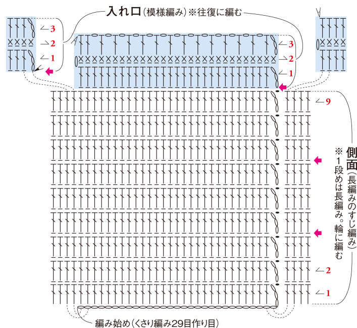
③「バネ口金ポーチ」の編み方記号図 【P100】
